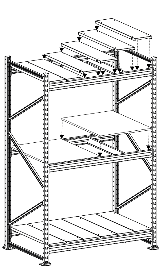
MPP 2,00m x 1,20m x 0,80m * 06 (seis) prateleiras metálicas por nível. * 02 (duas) prateleiras de MDP por nível.
