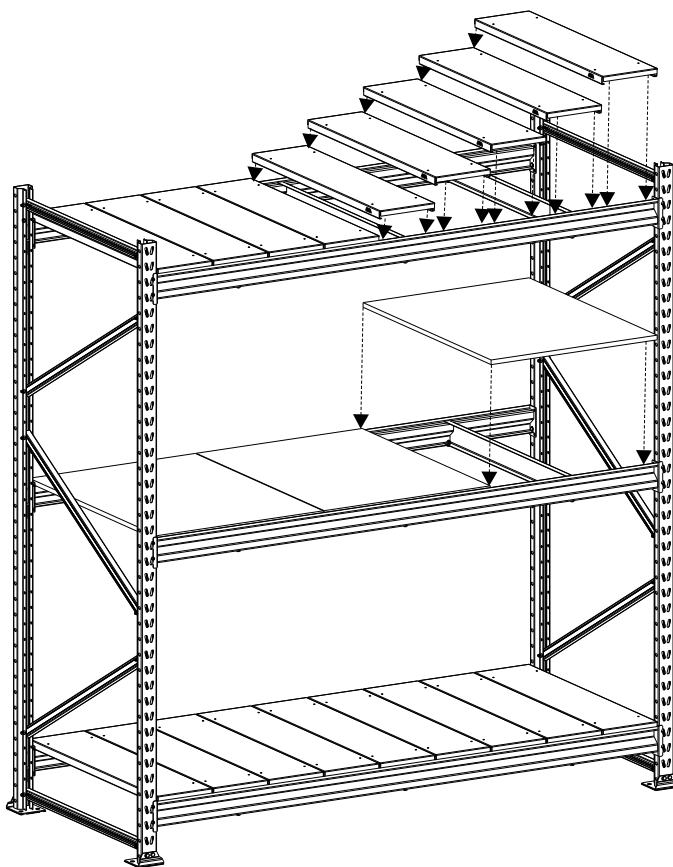
MPP 2,00m x 1,80m x 0,80m * 09 (nove) prateleiras metálicas por nível. * 03 (três) prateleiras de MDP por nível.
