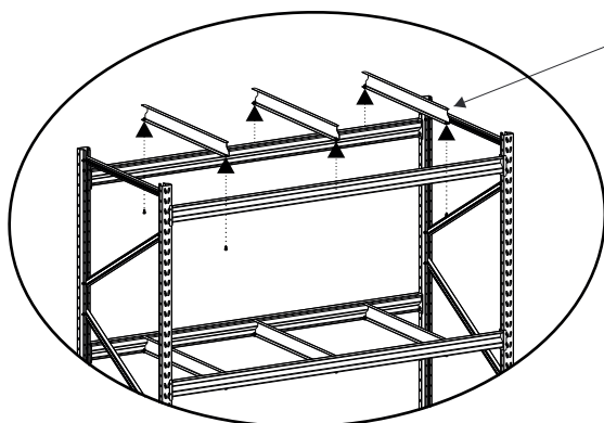
2,00m x 1,80m x 0,80m 03 (três) travessas por plano.
