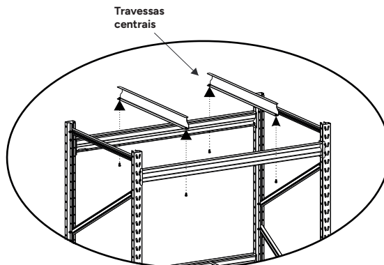
2,00m x 1,20m x 0,80m 02 (duas) travessas por plano.
